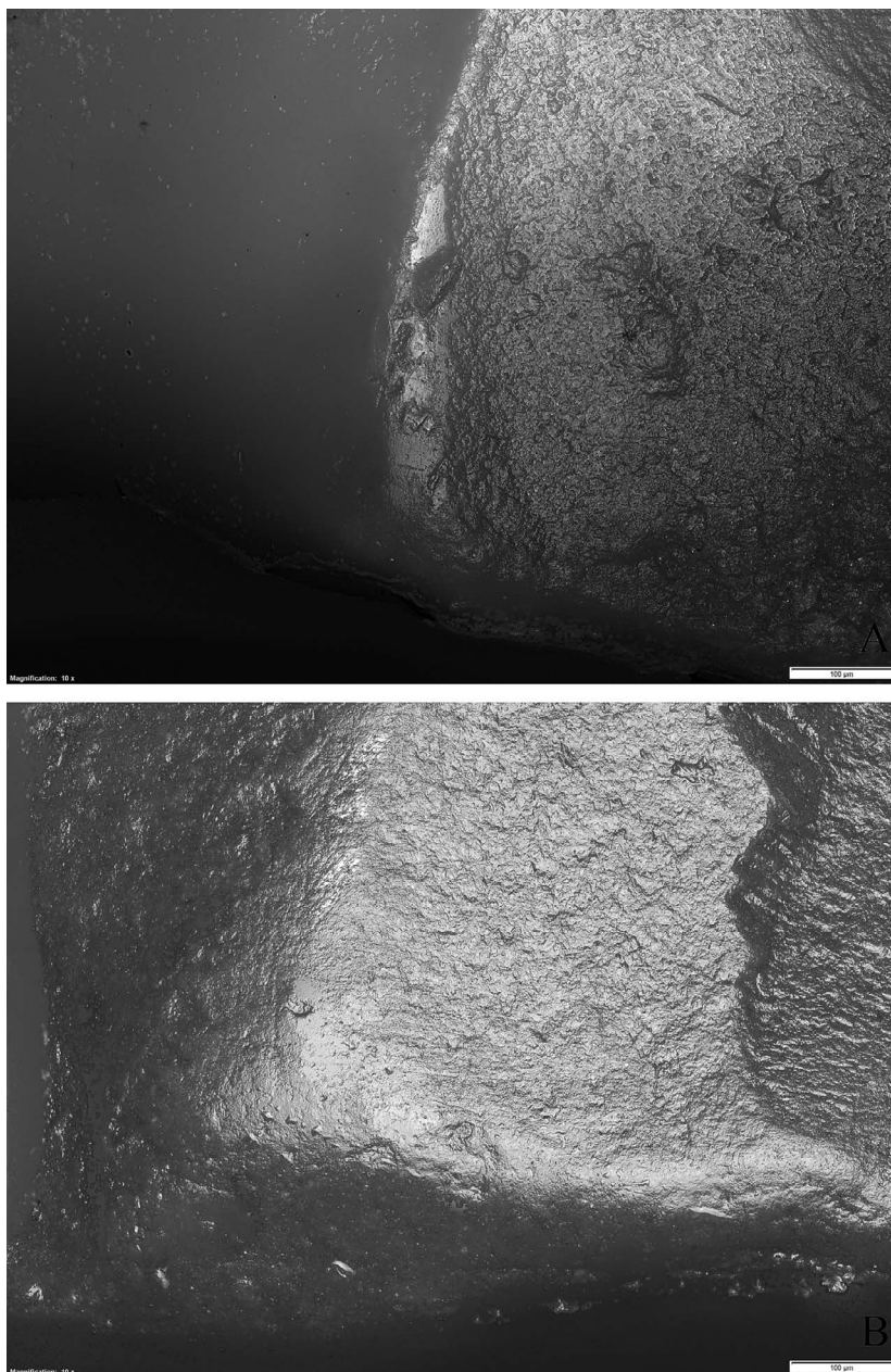
Obr. 17. Ostře ohraničené plochy plochého jasného lesku způsobeného otěrem tvrdým materiálem (pravděpodobně dřevem ratišť okolních šípů) při zvětšení 200x; uvedené měřítko 100 μm: A – projektil H10_01 dorzálně zprava, B – projektil H36_01 ventrálně zleva.
